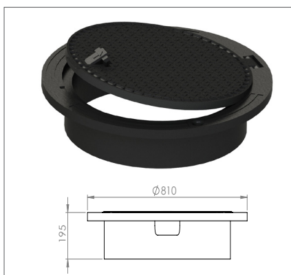
403428 Varitank dekselset, Rond klasse D gietijzer. Het dekselset is geheel van gietijzer en voorziet in een ronde kraag met een scharnierend deksel. De ronde kraag valt telescopisch over de Varitank schacht en is perfect geschikt om in een asfalt laag te verwerken, geheel is klasse D (zwaar verkeer) belastbaar.
