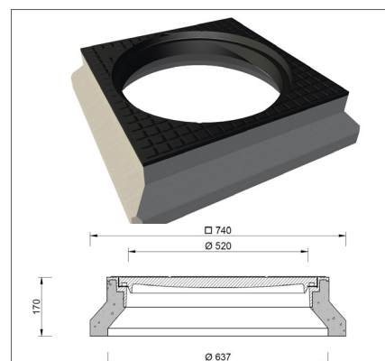
403426 Varitank dekselset vierkant klasse D400 + drukverdeelplaat. Rondgietijzerendekselin vierkantdekselkader van gietijzer en beton. Dekselconstructie is verkeersklasse D (zwaar verkeer) en voorzien van een extra fundatieplaat van beton, deze biedt een ultieme bescherming van de put of tank tegen grote gewichtsbelasting.
